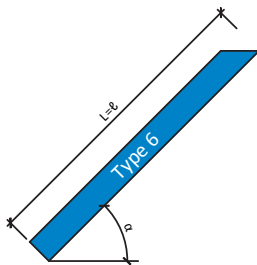
Horizontale afschuiving nok Toegelaten helling 32° tot 90°
