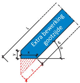
Verticale & horizontale afschuiving goot (basisafschuiving verticaal => verlenging z) Toegelaten helling 32° tot 58°
